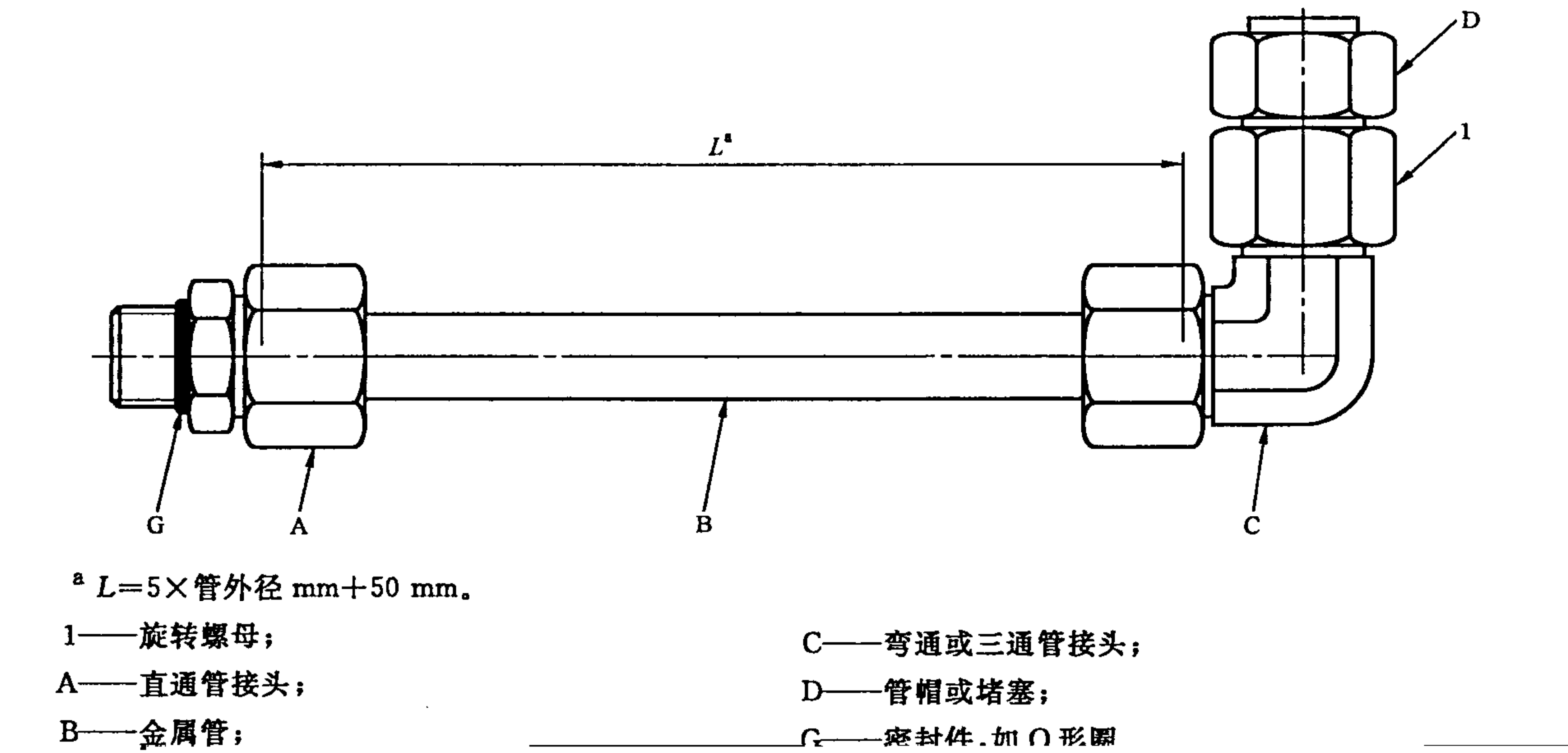
图 B.1 管连接试验总成——1 型
